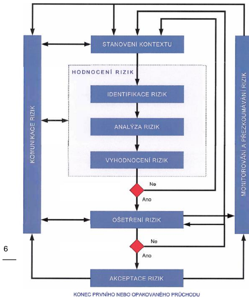
Obrázek 1 – ISO/IEC 27005: Proces řízení rizik
